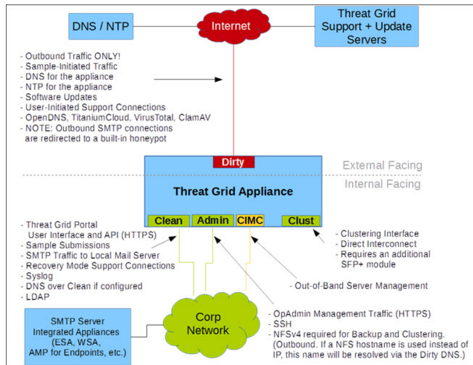
図 2: ネットワークインターフェイスの設定図
