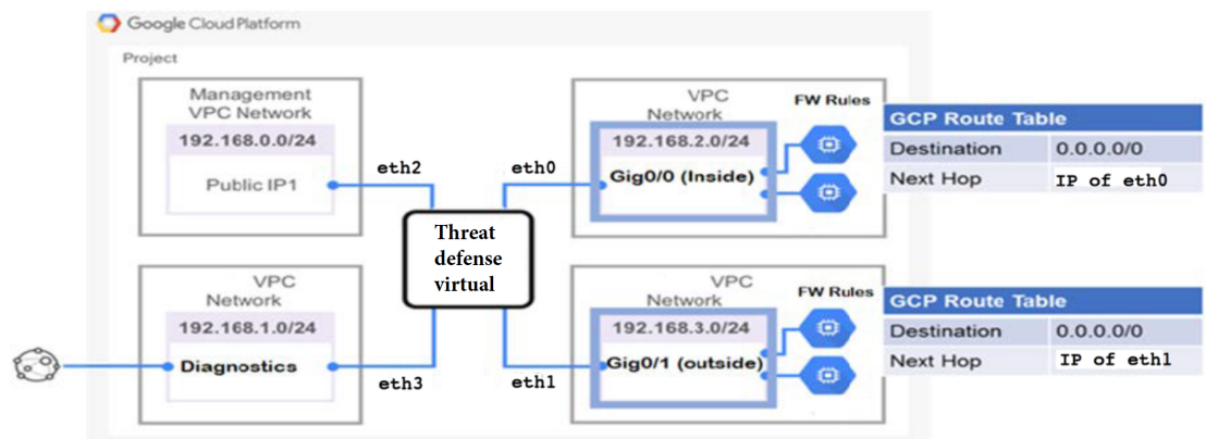
図 45: GCP 展開での Threat Defense Virtual の例
