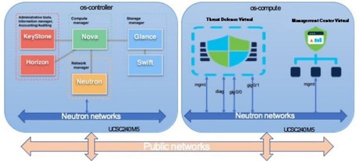
図 53: OpenStack で Threat Defense Virtual と Management Center Virtual を使用したトポロジーの例
