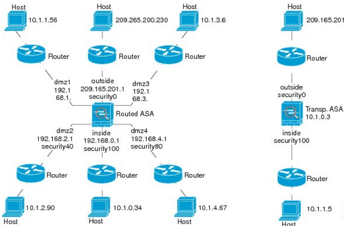
図 1: インターフェイス、ルータ、およびホストを含むネットワーク図
