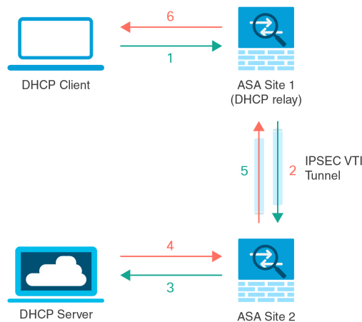
図 1: VTI を介した DHCP リレーサーバー
