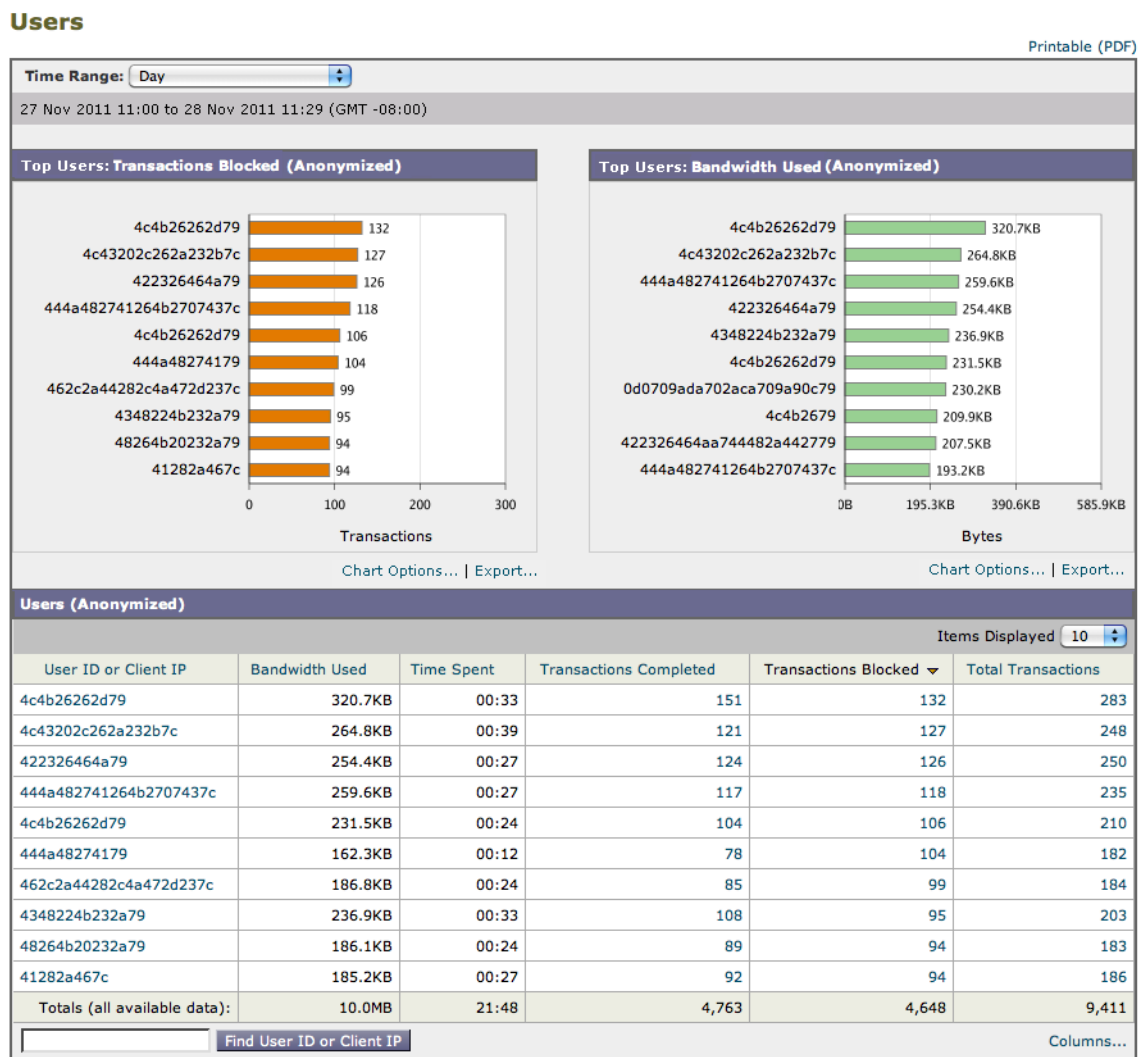
図 5-2 ユーザを匿名にしたレポートのページ
