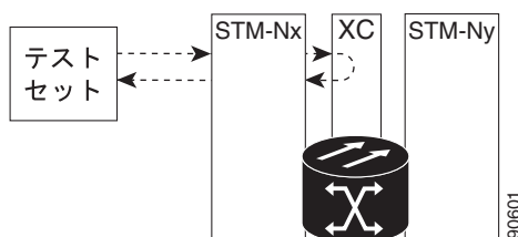
図 1-22 発信元 STM-N ポートでの XC ループバック
