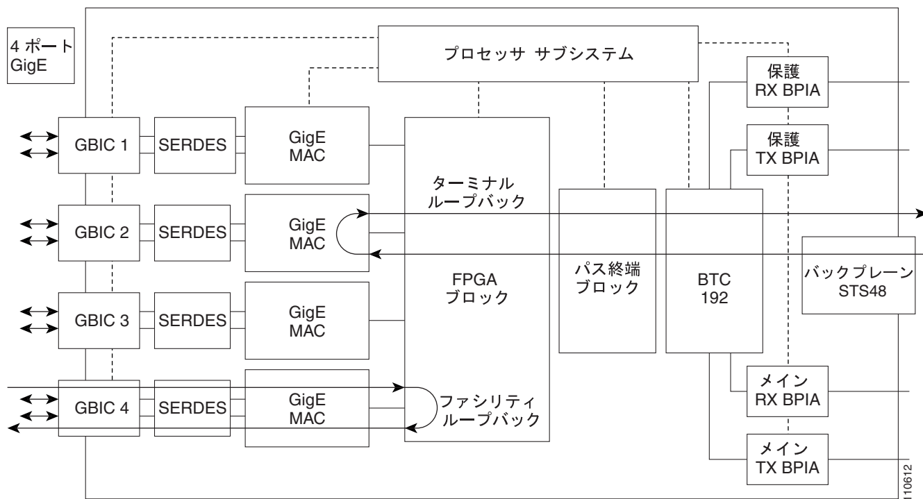
図 1-29 G シリーズポートでのターミナルループバック
