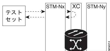
図 1-17 発信元 STM-N ポートでの XC ループバック
