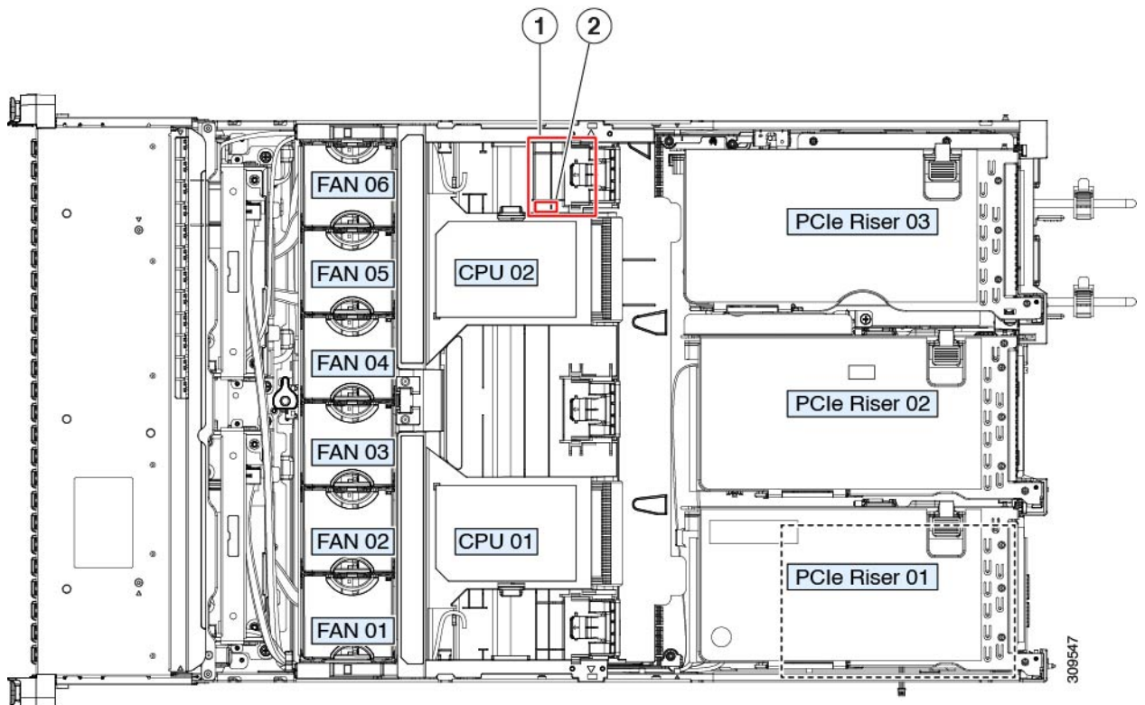
図 31: エアージャケット上の SuperCap ブラケット
