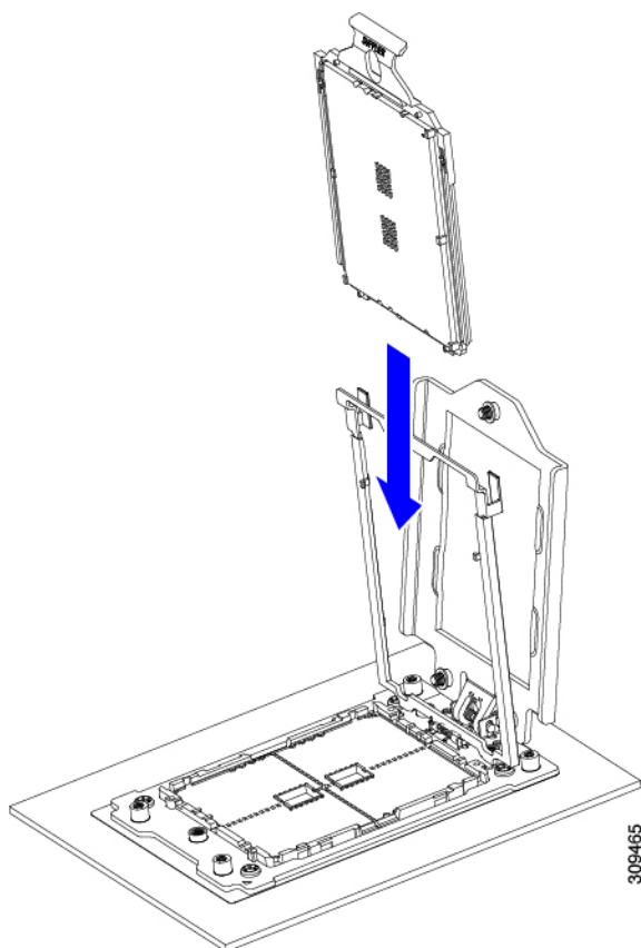
図 15: CPU をキャリアフレームに挿入します。
