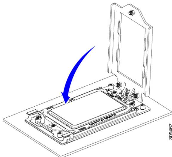
図 17: ソケットフレームの閉じ方
