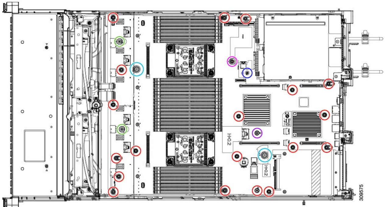
図 35: HX C245 M6 PCBA を取り外すネジの位置
