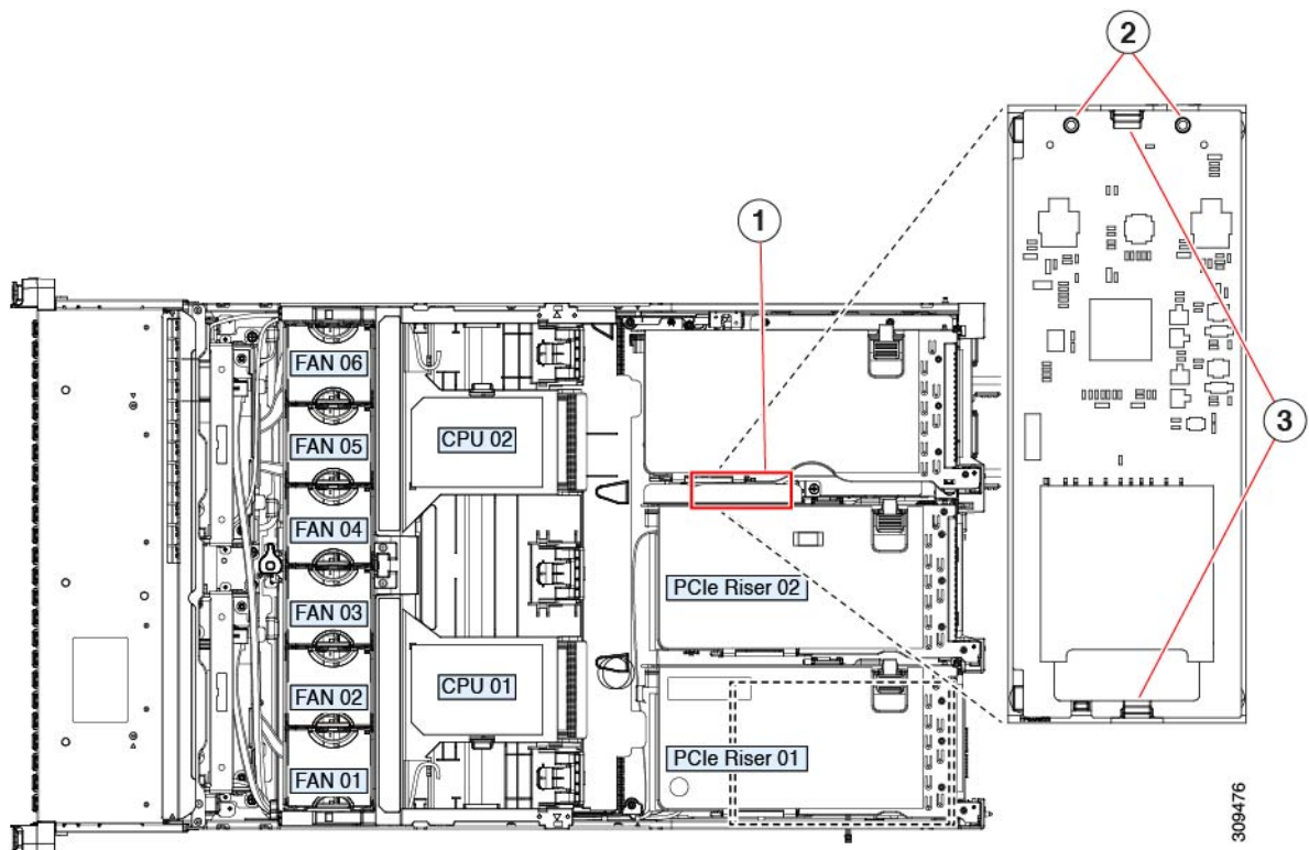
図 22: ミニストレージモジュールキャリアソケット
