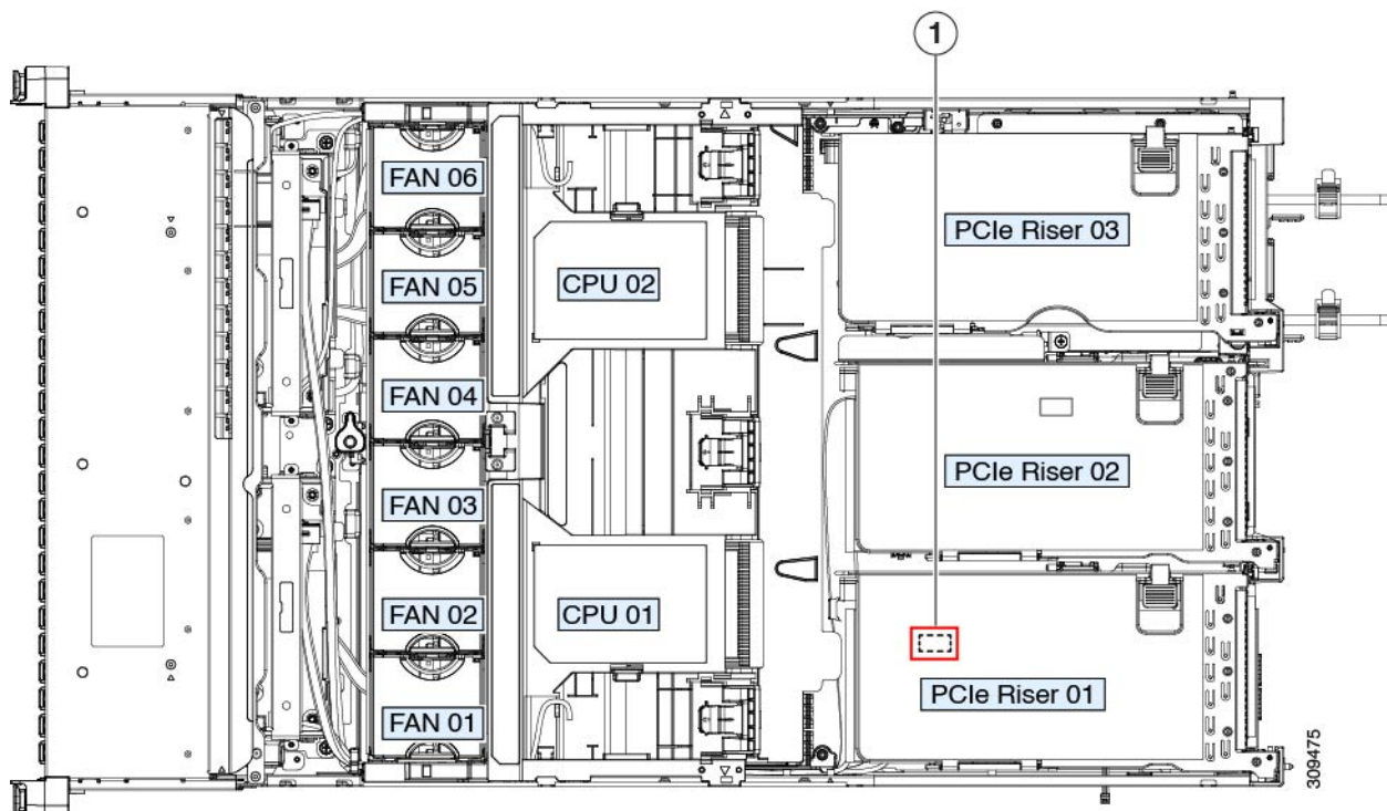
図 23: 内部 USB ポートの場所
