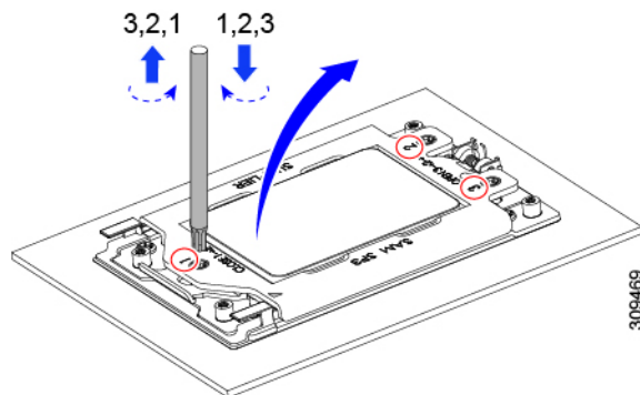
図 11: ソケット フレーム ネジをゆるめる
