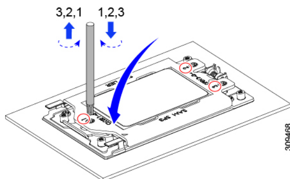
図 18: ソケットフレームの閉じ方
