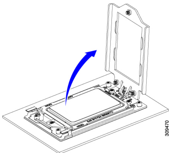
図 12: ソケットフレームを開く
