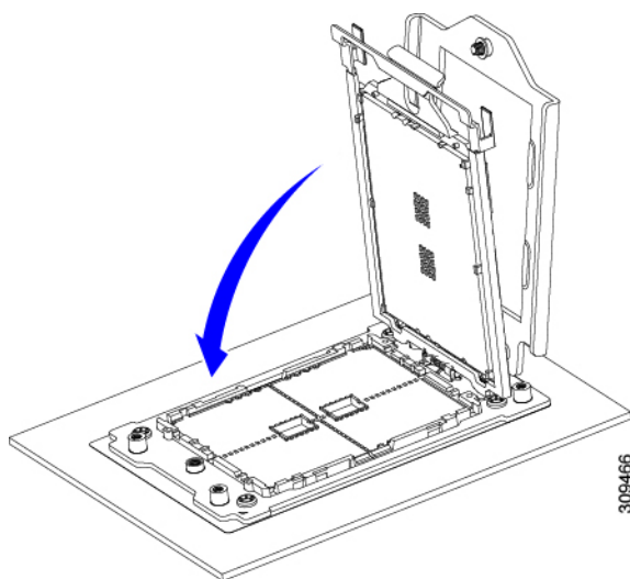
図 16: レールフレームを閉じる
