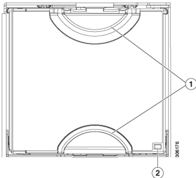
図 9: ファン モジュールの上面図
