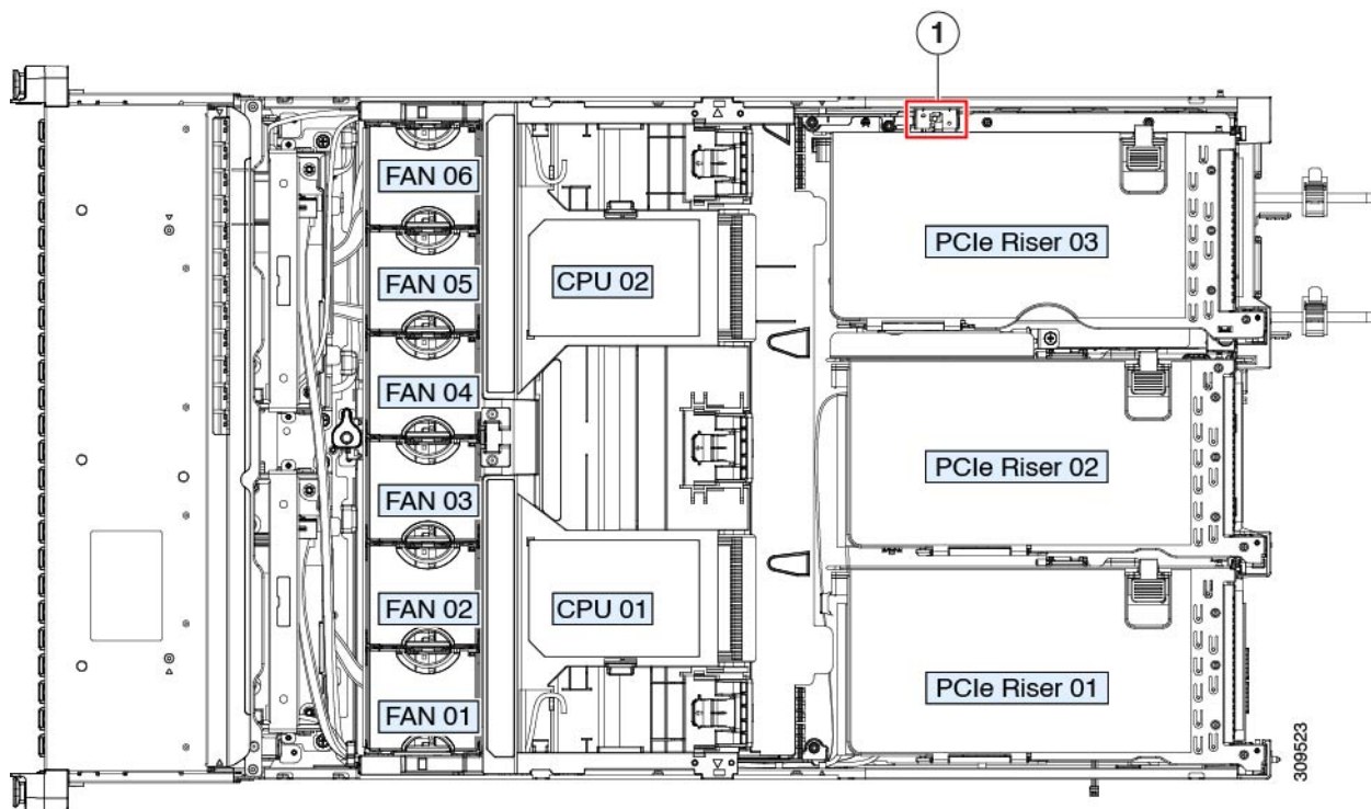
図 33: シャーシ侵入スイッチの交換
