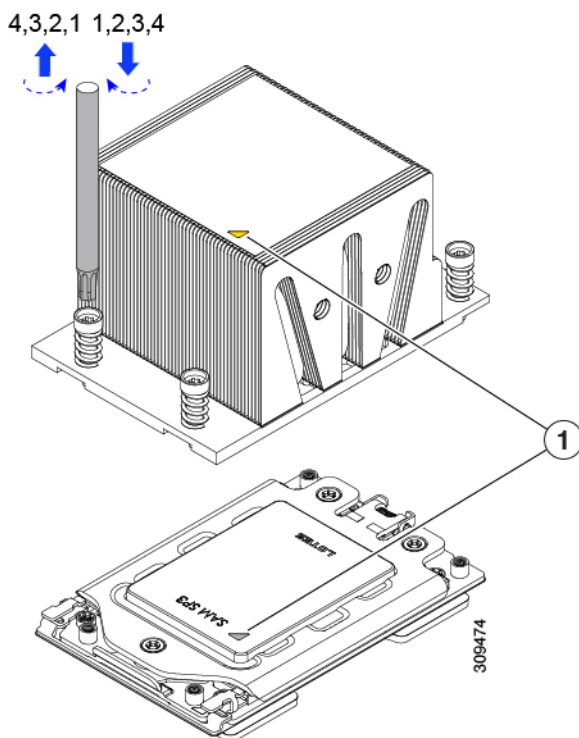
図 20: ヒートシンク配置マーク
