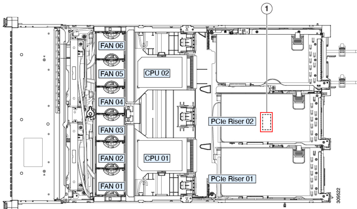
図 34: TPM ソケットの場所
