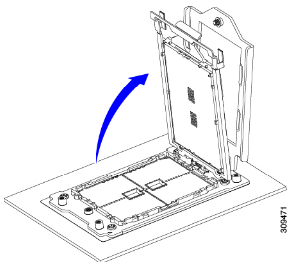
図 13: レールフレームを開く
