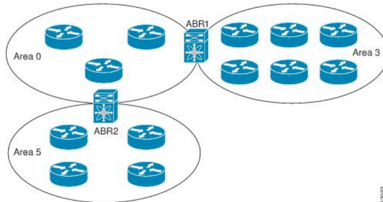
図 19: OSPFv3 エリア
