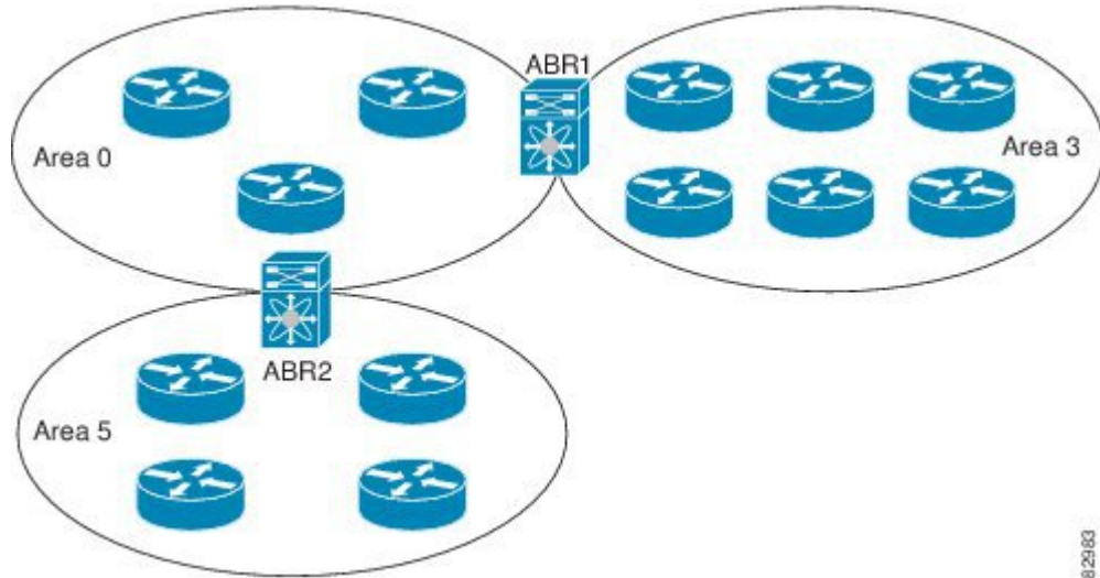
図 2: OSPFv2 エリア
