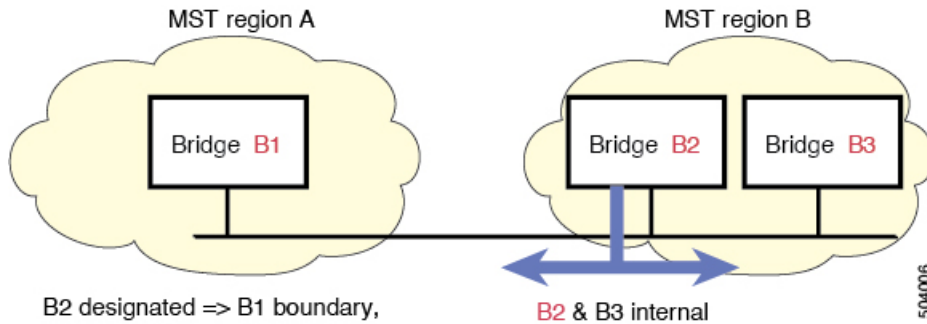
Figure 2: MST 境界ポート
