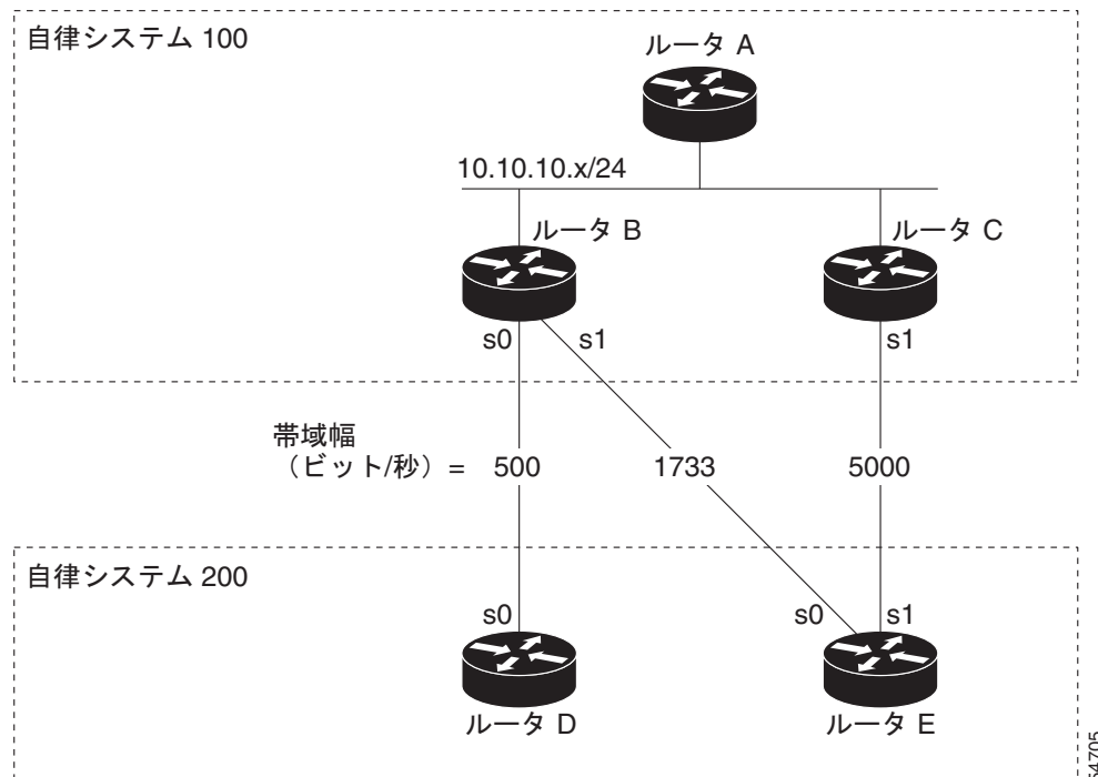
図 1 BGP リンク帯域幅の設定
