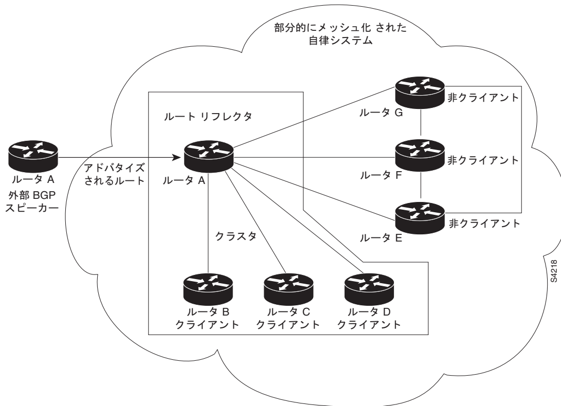
図 3 より複雑な BGP ルート リフレクタのモデル
