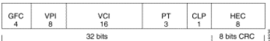
図 1 : ATM ユーザ ネットワーク インターフェイス ( UNI ) セル ヘッダーの形式
