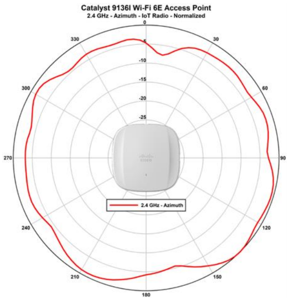
図 2. アンテナのプロファイル
