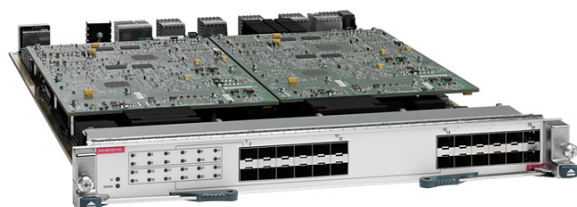
図 1. Cisco Nexus 7000 M2 シリーズ XL オプション 24 ポート 10 ギガビット イーサネット モジュール
