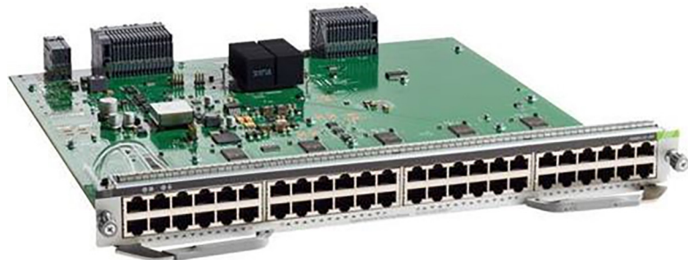
図 10. Cisco Catalyst 9400 シリーズ 48 ポート 10/100/1000 (RJ-45) ラインカード (C9400-LC-48T)
