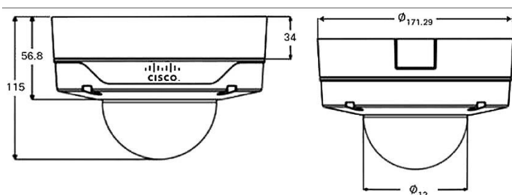
図 1. Cisco Video Surveillance 7530PD IP カメラの寸法
