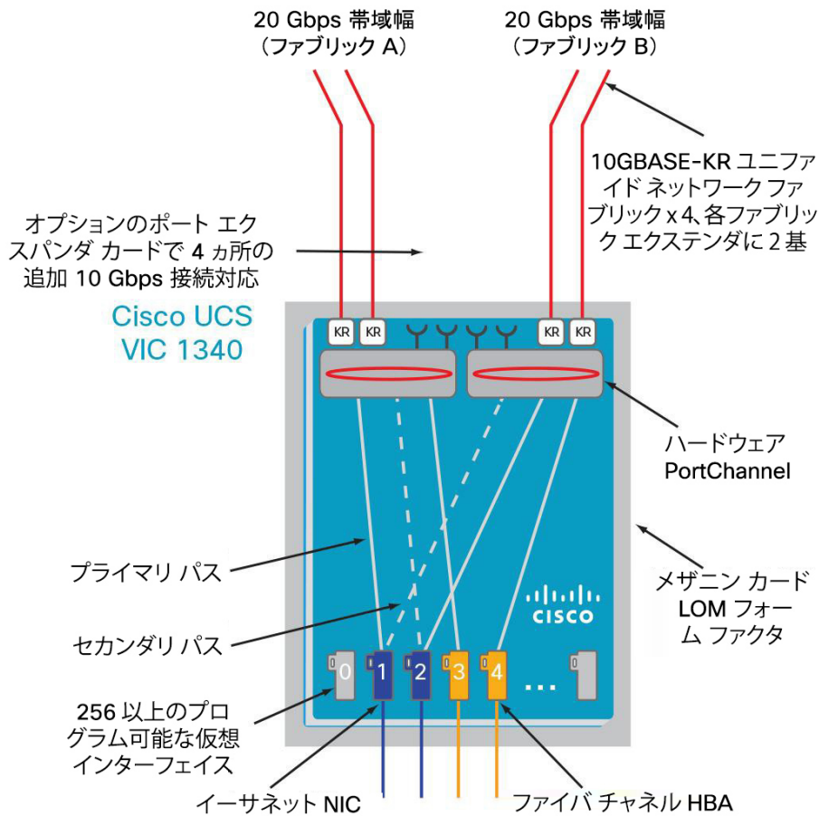
図 2 Cisco UCS VIC 1340 アーキテクチャ
