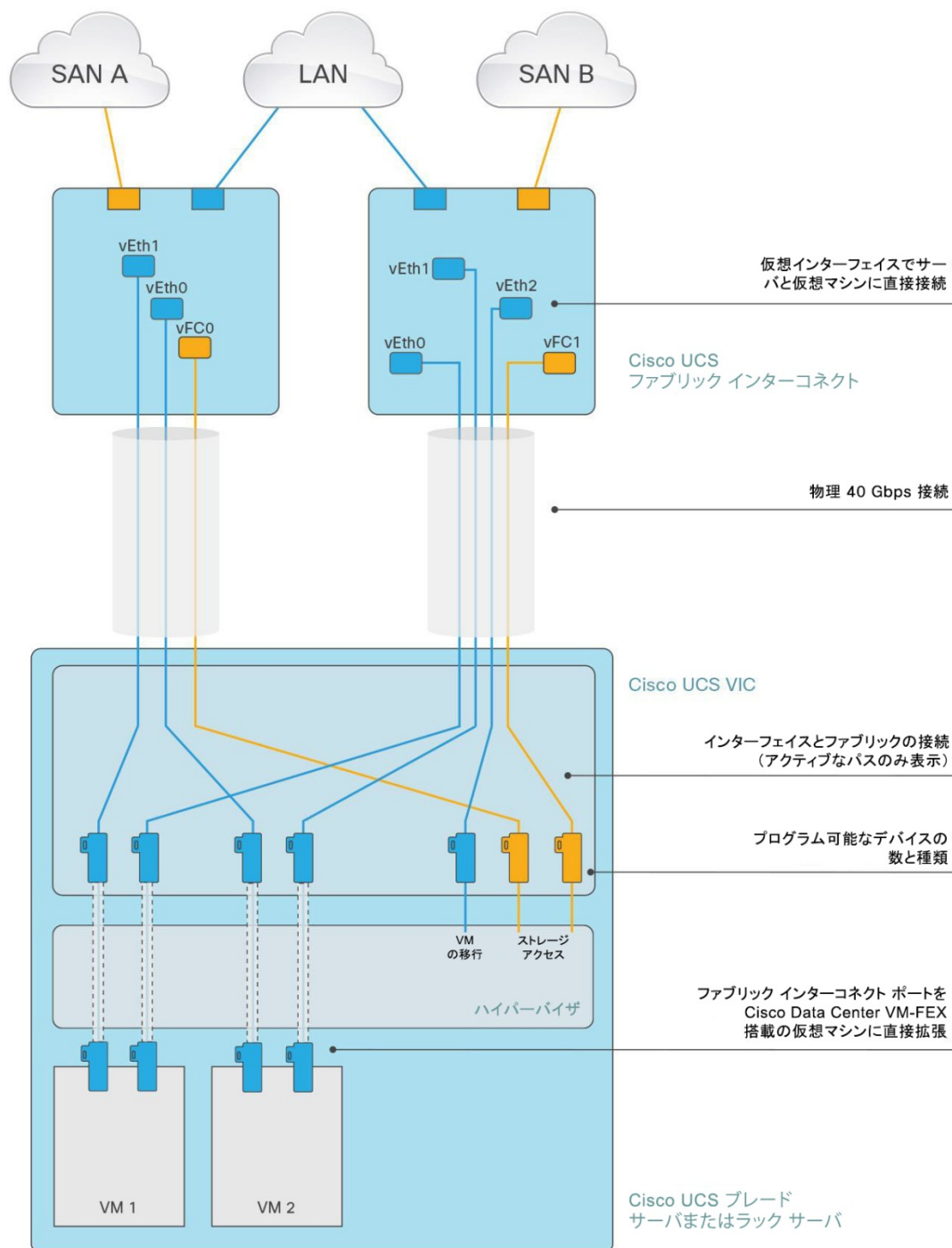
図 3 Cisco UCS VIC 1340 での Cisco Data Center VM-FEX
