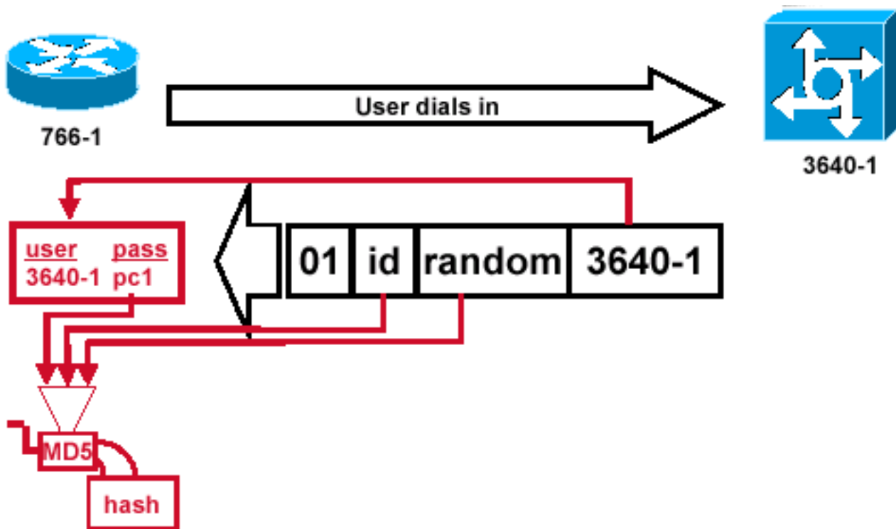
Figura 4: Recepción y procesamiento MD5 del paquete de desafío del par
