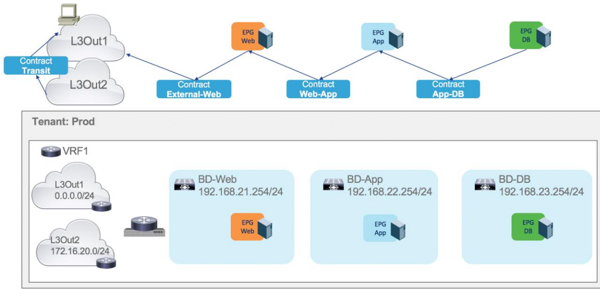
Figure 2. Tenant topology
