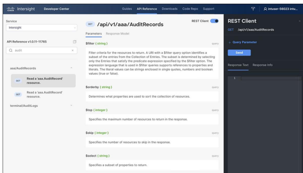
Figure 58. API browser
