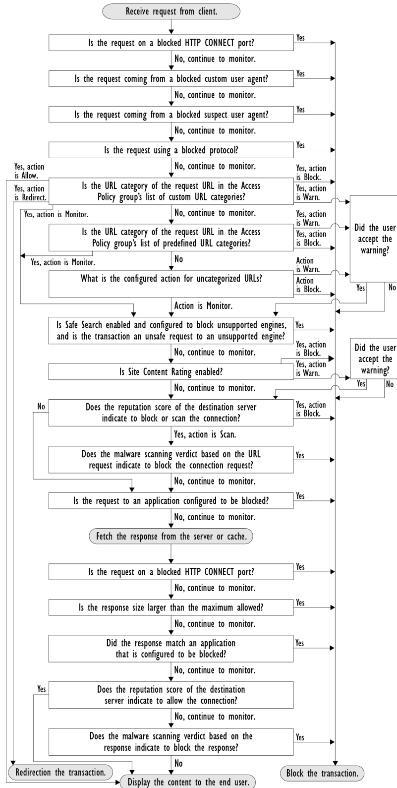
図 10-4 アクセスポリシーのアクションの適用
