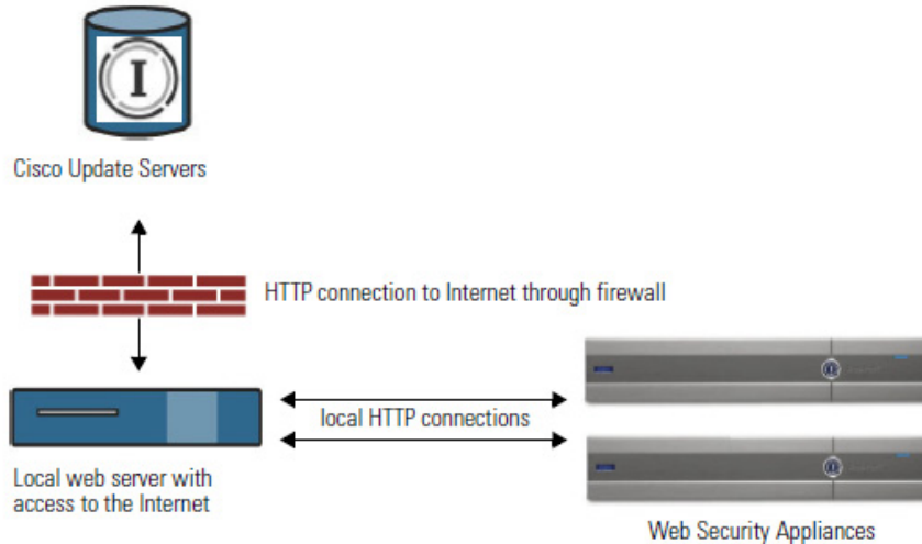
図 22-1 ローカル サーバからのアップグレード
