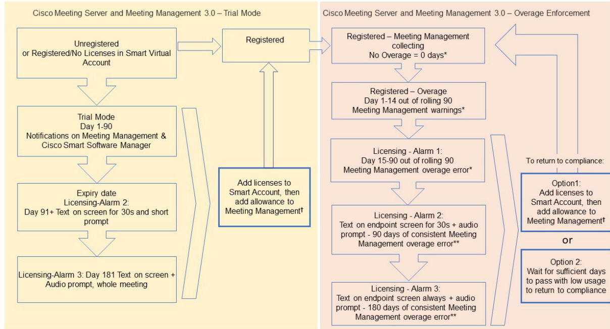
図 21 : Cisco Meeting Server と Cisco Meeting Management スマート ライセンスの強制フロー
