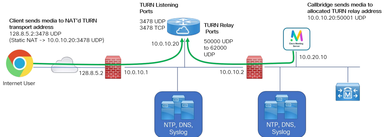
図 8 : TURN サーバーリレーの例
