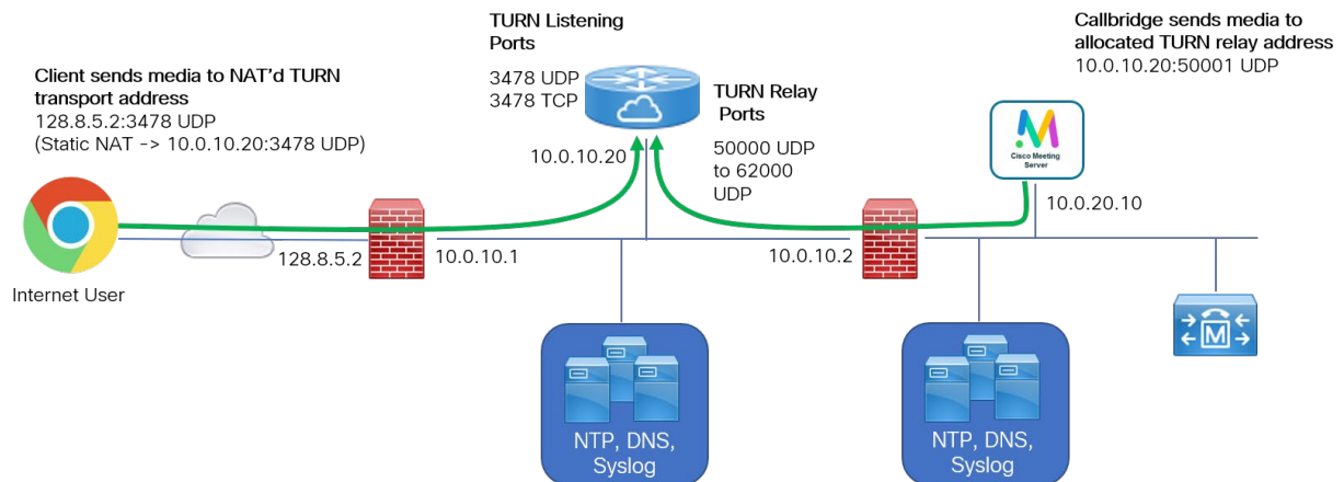
図 9 : UDP を使用した TURN のサンプル図
