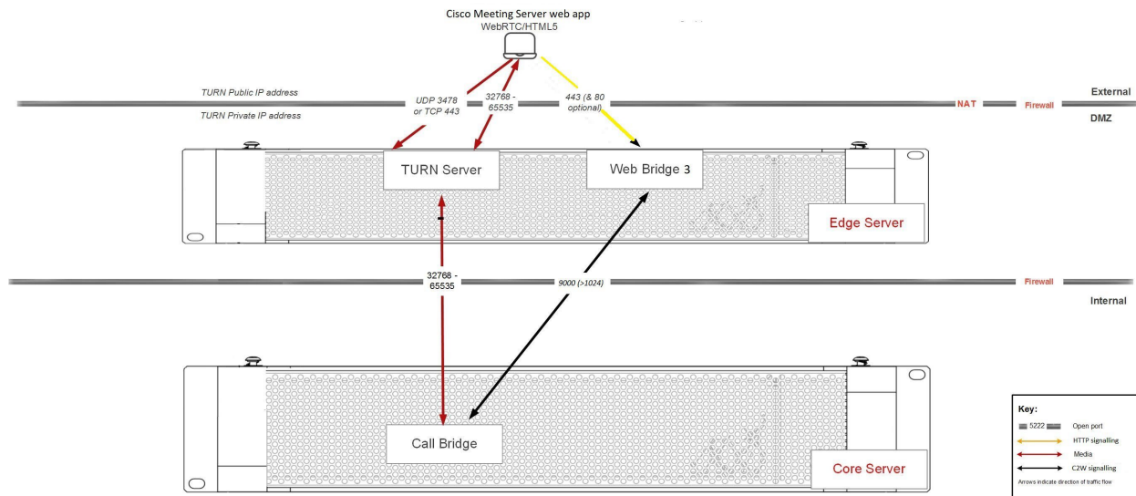
図 17 : Web アプリポートの使用法
