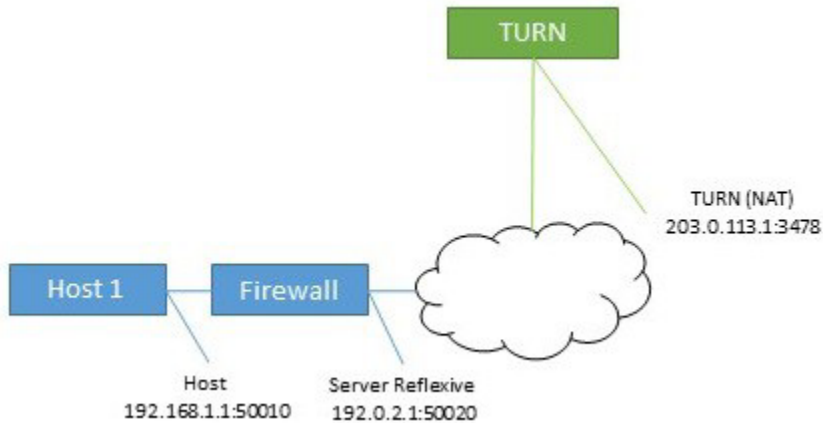
図 26 : サーバー再帰候補
