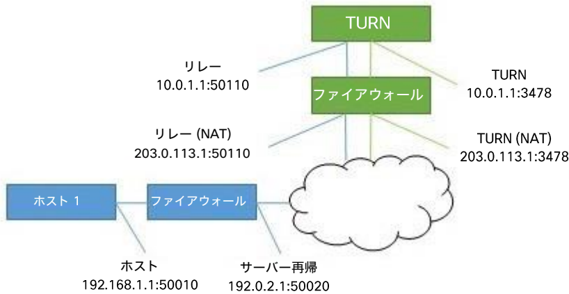
図 27 : リレー候補
