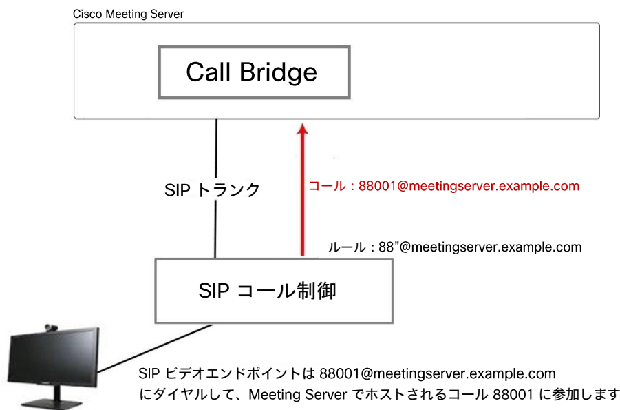
図 11 : Meeting Server でホストされたコールを呼び出す SIP ビデオエンドポイントの例
