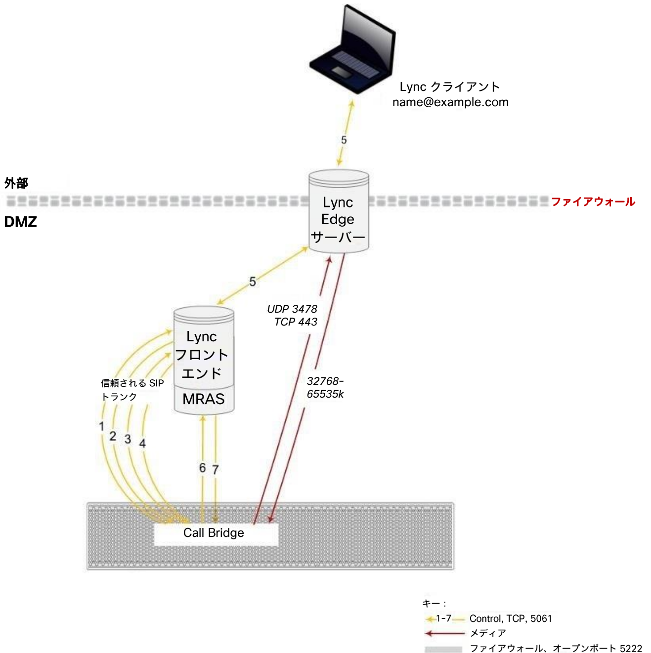
図 15 : Lync Edge サーバーへの Call Bridge のコールフロー
