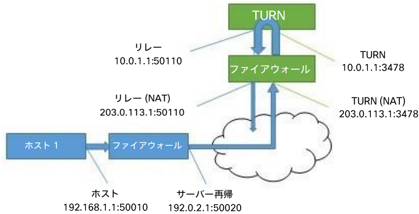
図 29 : 遠端へパケットを送信するホスト
