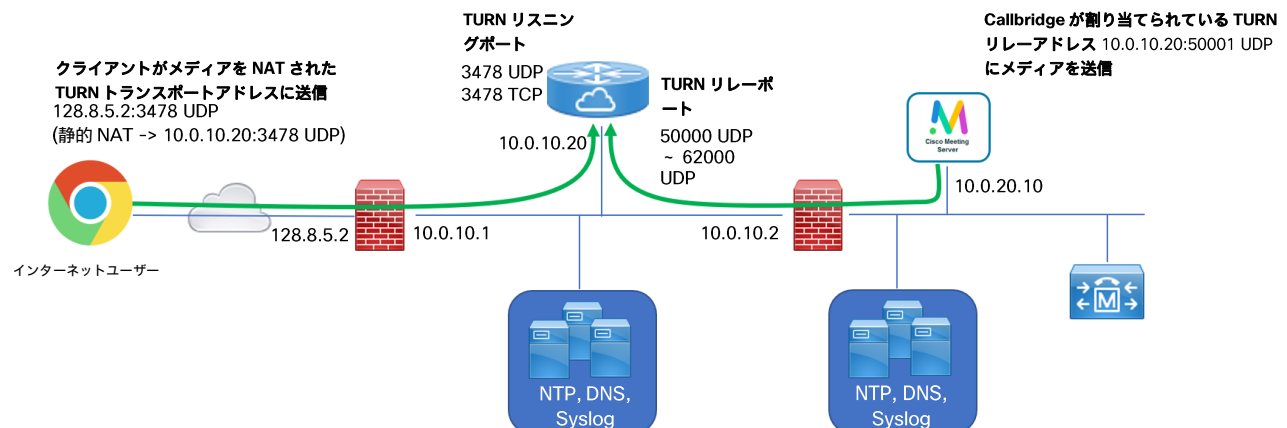
図 8：UDP を使用した TURN のサンプル図
