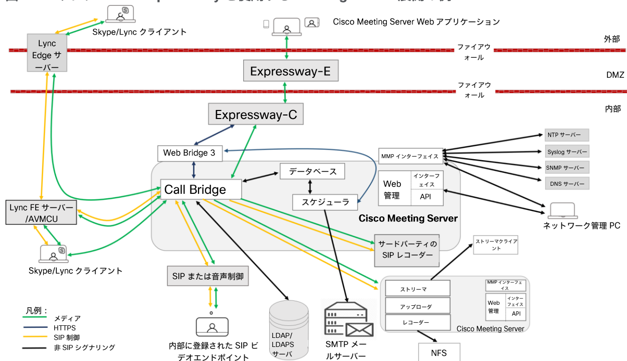
図 6 : エッジに Cisco Expressway を使用する Meeting Server 展開の例
