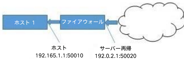
図 26 : NAT を実行するファイアウォールの背後にあるホストの影響
