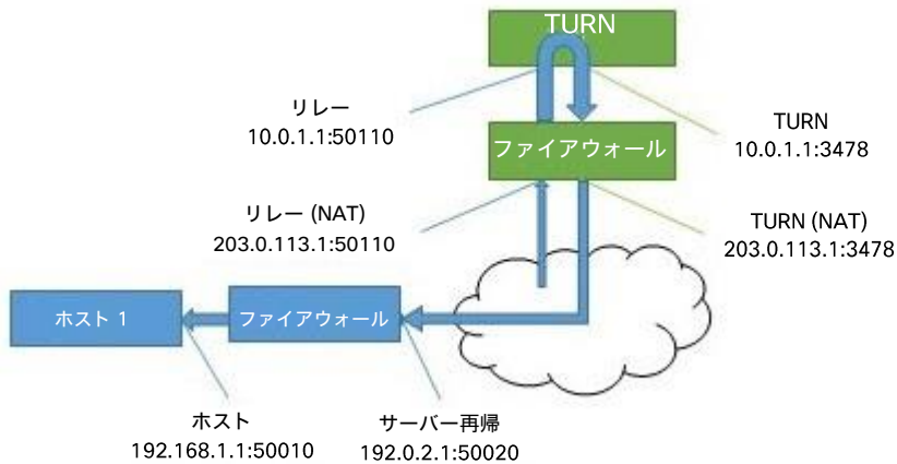
図 28 : TURN サーバがホストにリレーアドレスを返す
