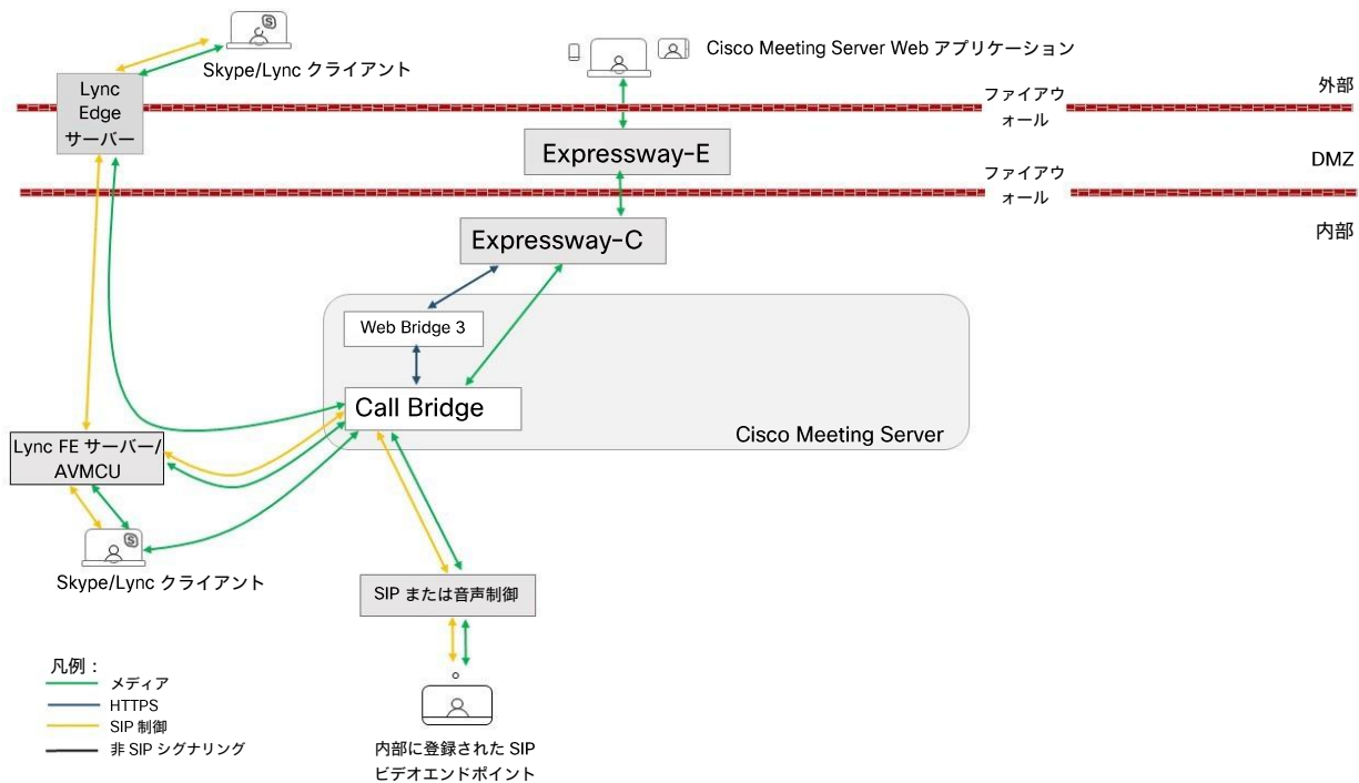
図 10：ダイアルプラン構成の展開例
