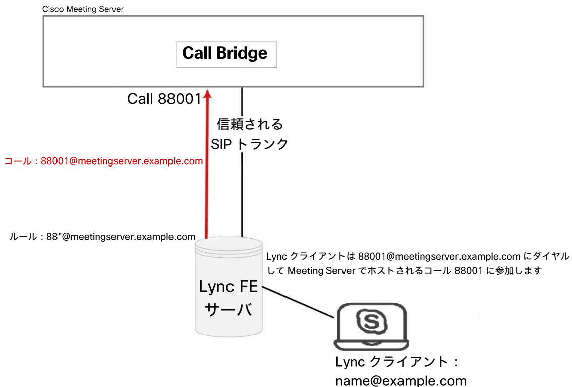
図 12 : Meeting Server でホストされた会議に発信する Lync クライアントの例
