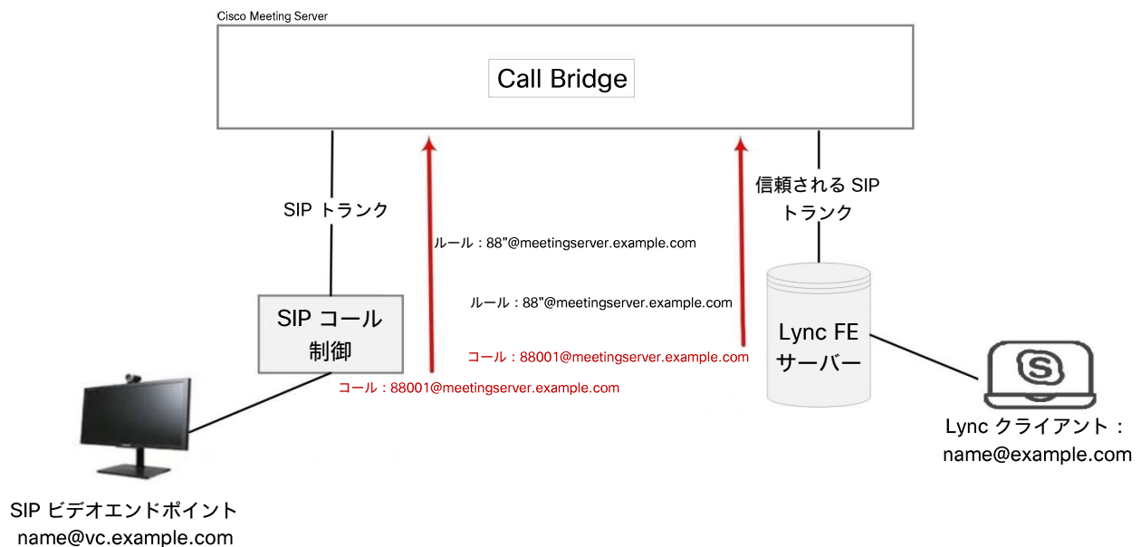
図 13 : Meeting Server でホストされた会議に発信する SIP ビデオエンドポイントと Lync クライアントの例
