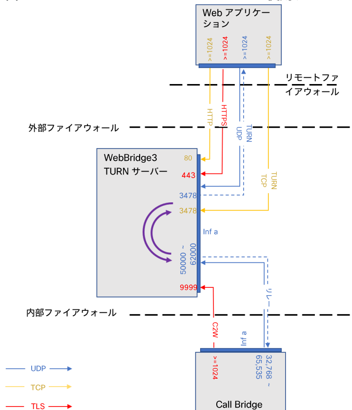
図 9：TURN 3478 UDP または 3478 TCP を使用する Web アプリ
