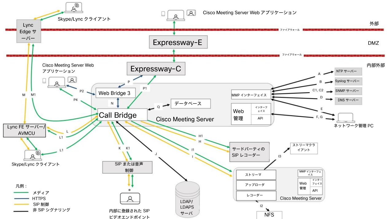
図 23 : DMZ 内の Expressway と組み合わせたサーバ展開で開く必要があるポート
