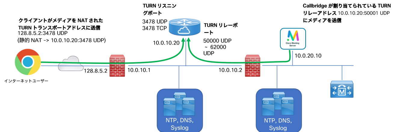
図 2 : Meeting Server Edge TURN サーバーの例
