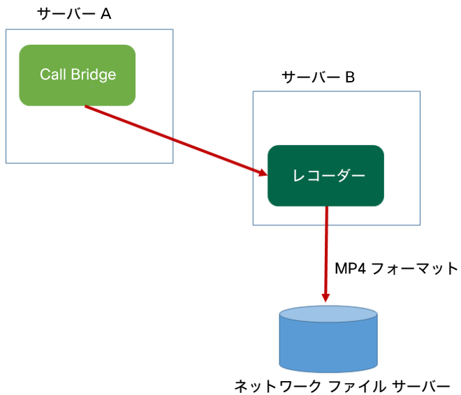
図 17：録画に許可されている展開：リモートモード
