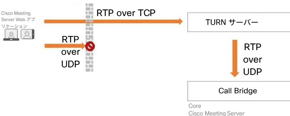
図 7 : TCP および UDP をサポートする TURN サーバ
