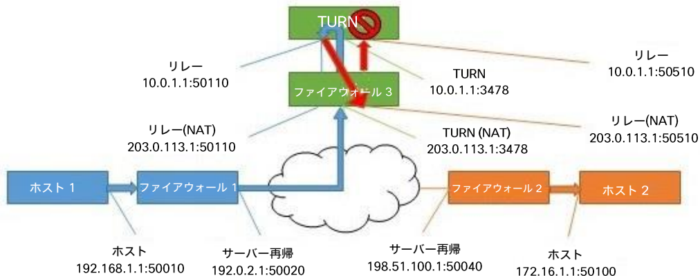
図 31 : リレー間のパスを使用したホスト間のメディアパス (NAT あり)
