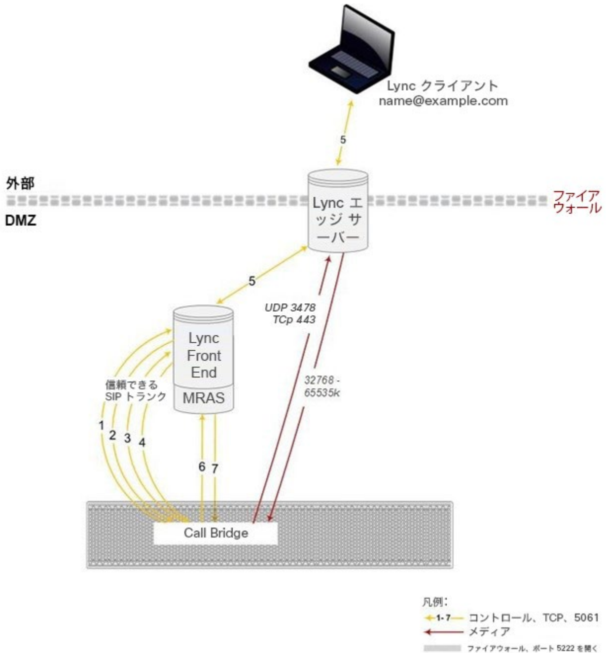
図 15 : Lync Edge サーバーへの Call Bridge のコールフロー
