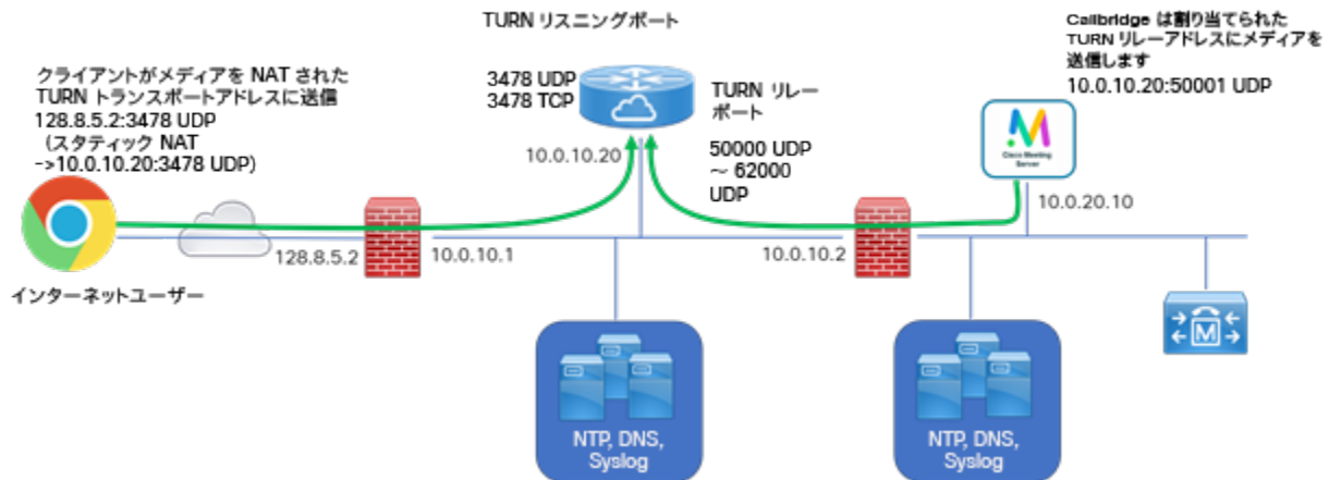
図 2 : Meeting Server Edge TURN サーバーの例
