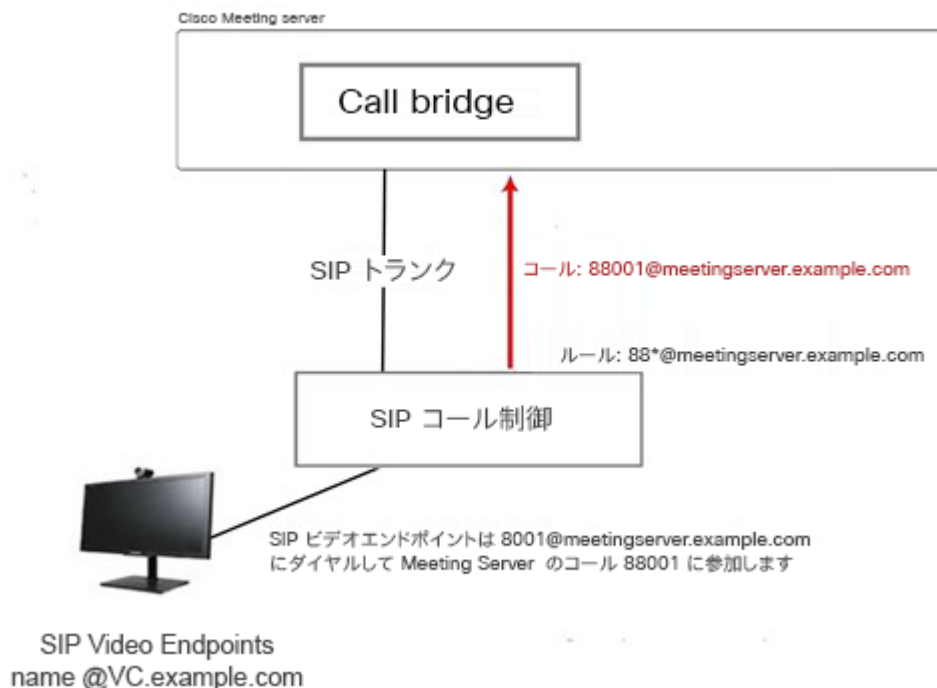
図 11 : Meeting Server でホストされたコールを呼び出す SIP ビデオエンドポイントの例
