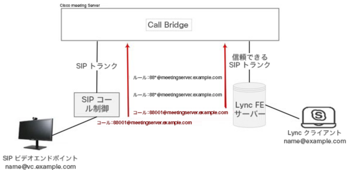
図 13 : Meeting Server でホストされたミーティングに発信する SIP ビデオエンドポイントと Lync クライアントの例
