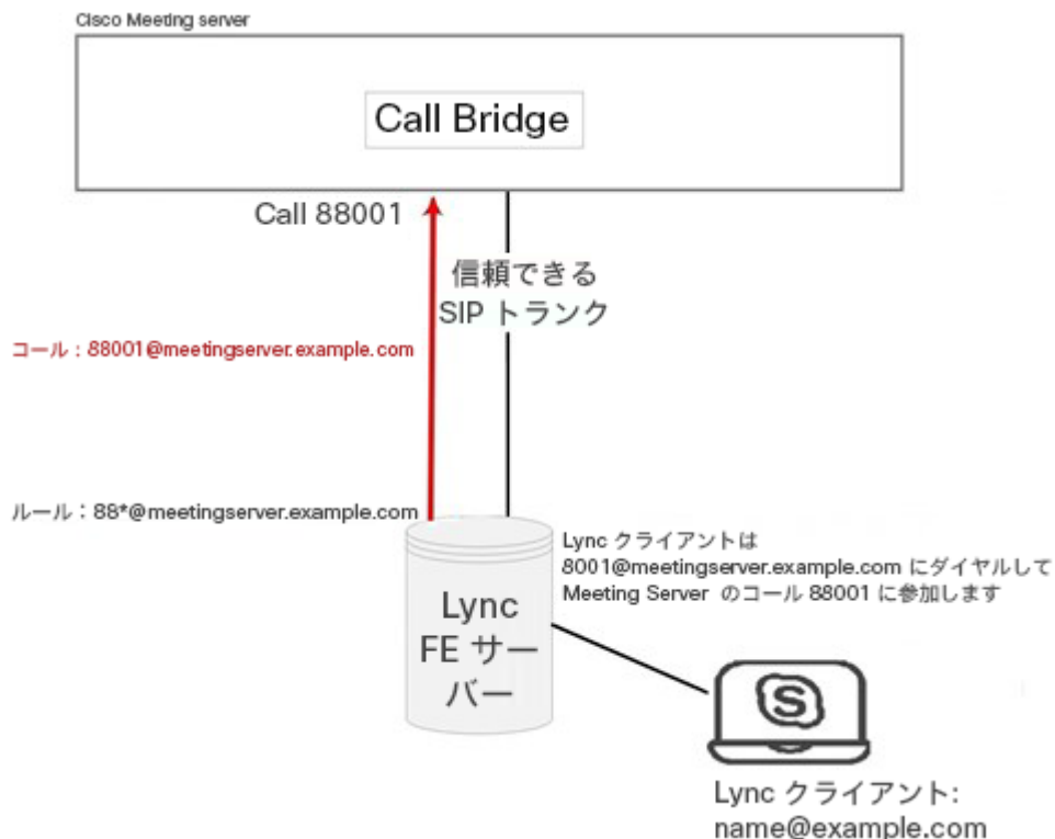
図 12 : Meeting Server でホストされた会議に発信する Lync クライアントの例
