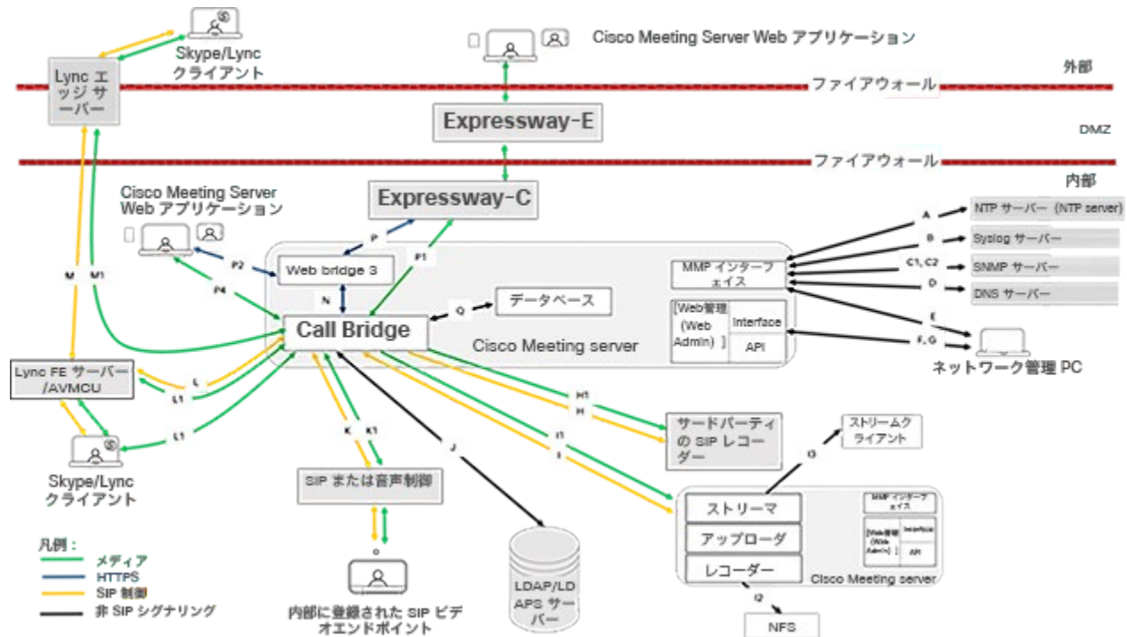
図 23 : DMZ 内の Expressway と組み合わせたサーバー展開で開く必要があるポート
