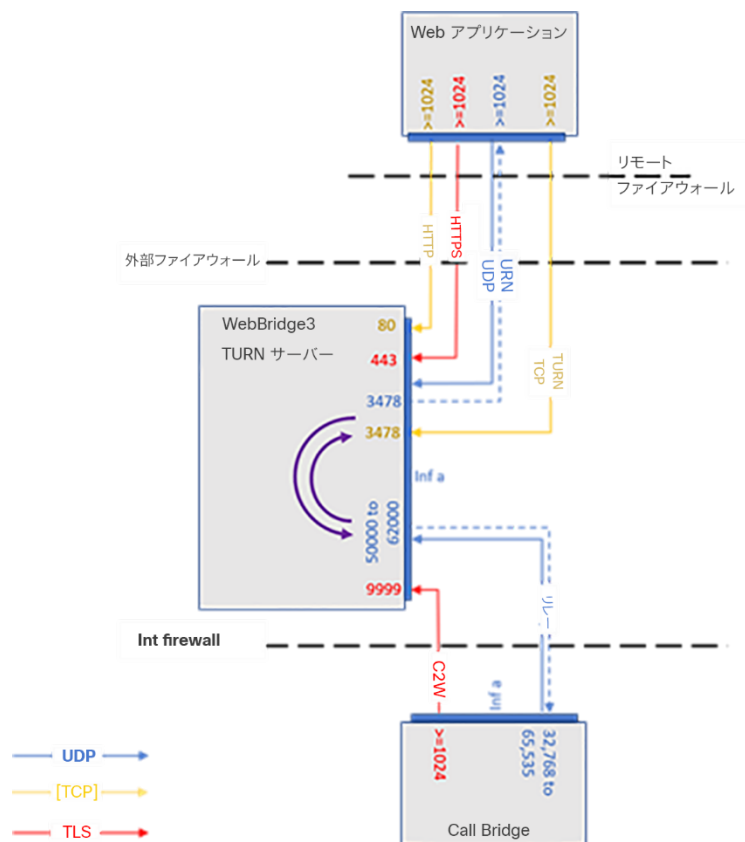
図 9 : TURN 3478 UDP または 3478 TCP を使用する Web アプリ
