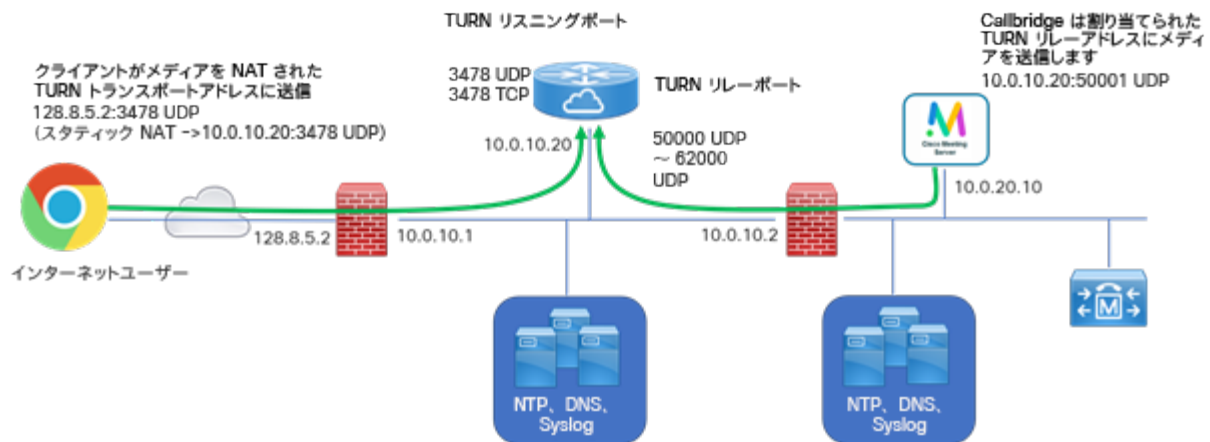
図 8 : UDP を使用した TURN のサンプル図
