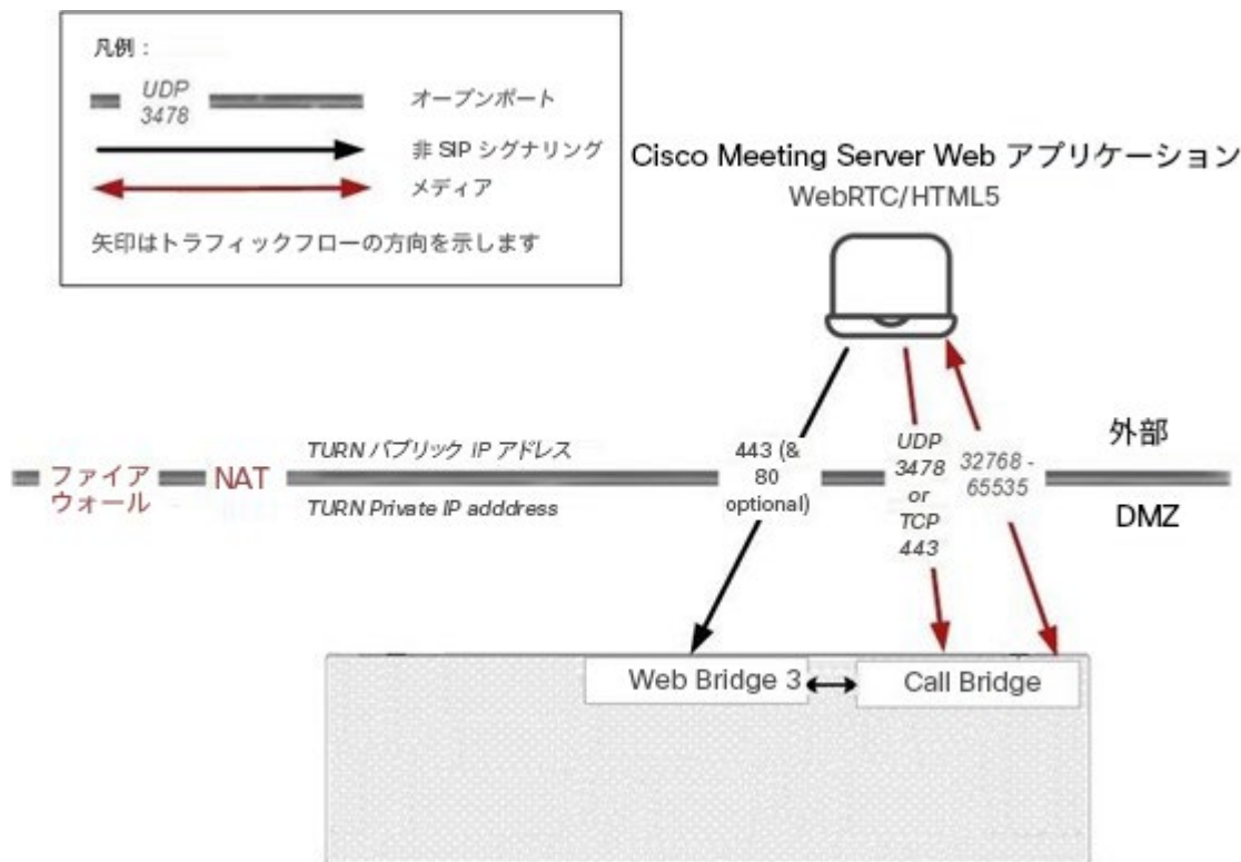
図 16 : Web アプリポートの使用方法
