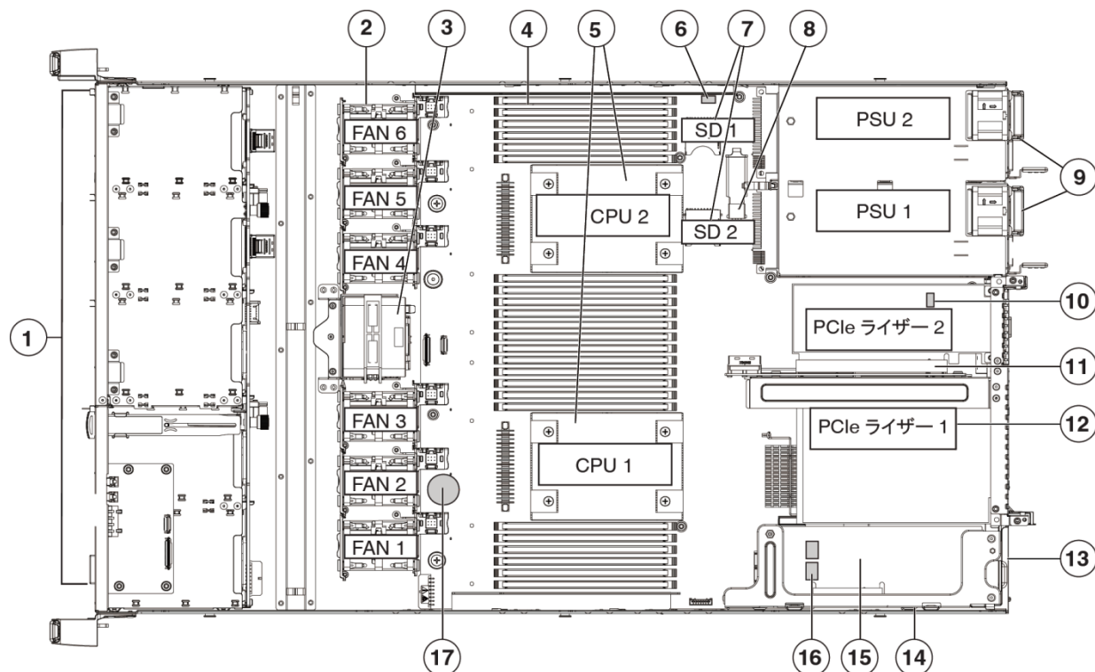
図 6 上部カバーを外した C220 M4 SFF
