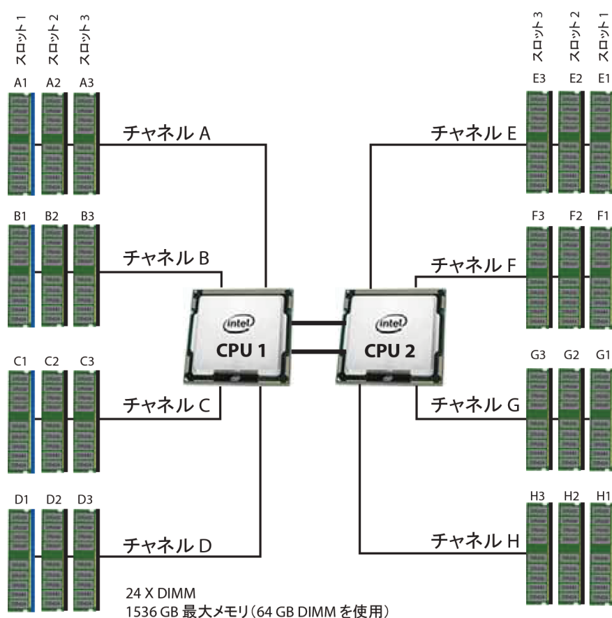
図 4 C220 M4 SFF メモリ構成
