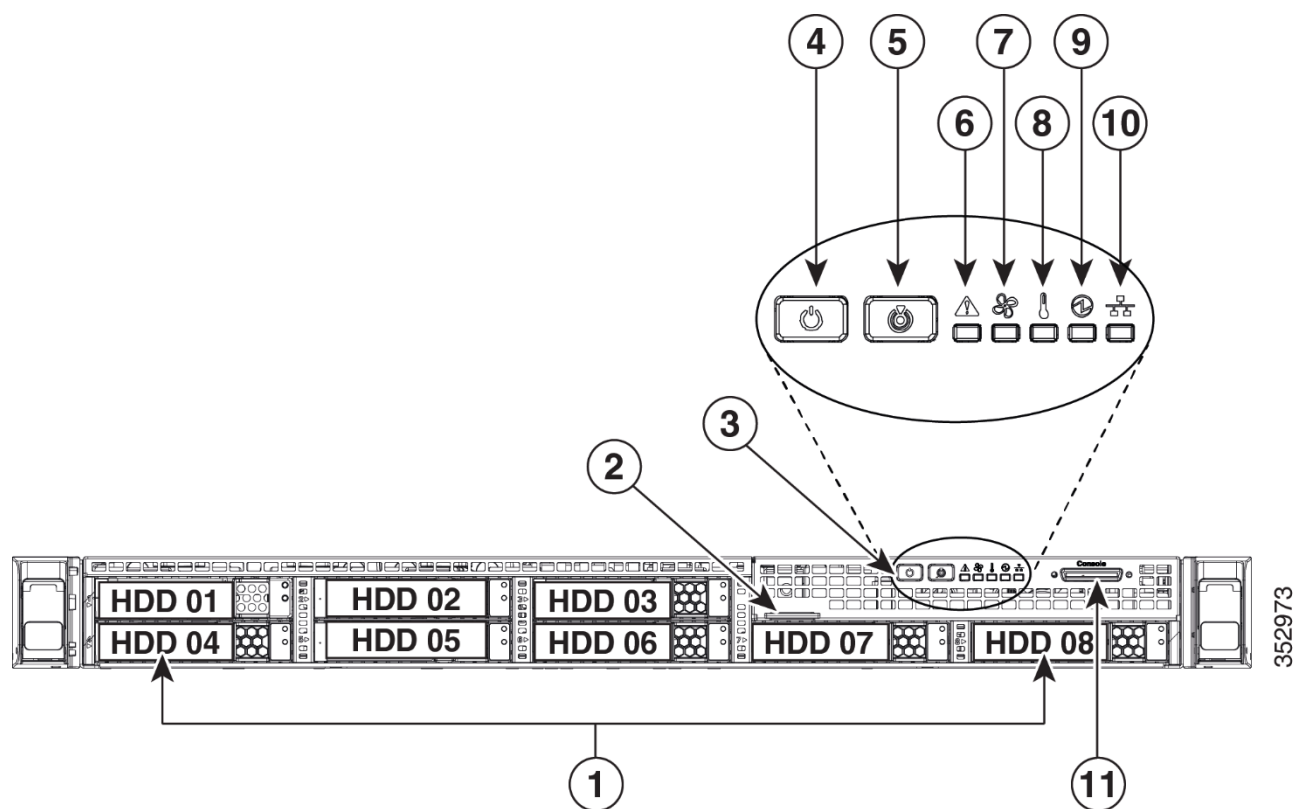
図 2 シャーシ正面図
