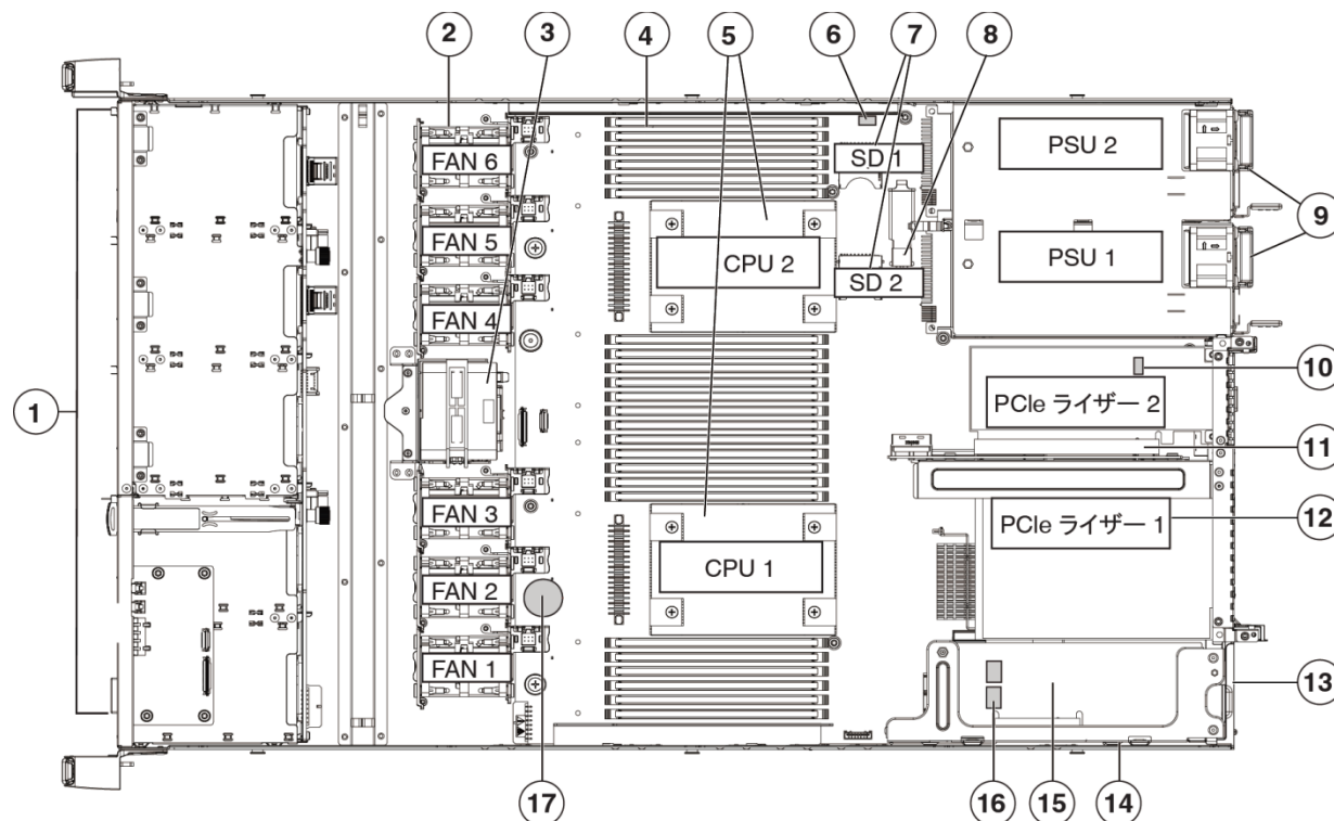
図 16 マザーボード上の USB ポート、SD ポート、RAID カード SuperCap の位置
