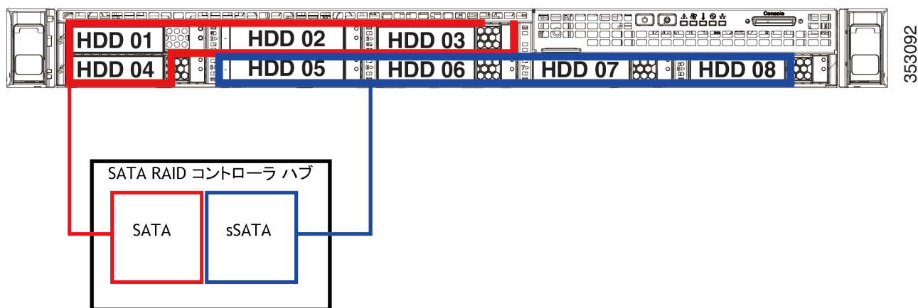
図 10 組み込み RAID コントローラの RAID グループ
