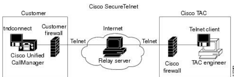
圖 26: Cisco Secure Telnet 系統
